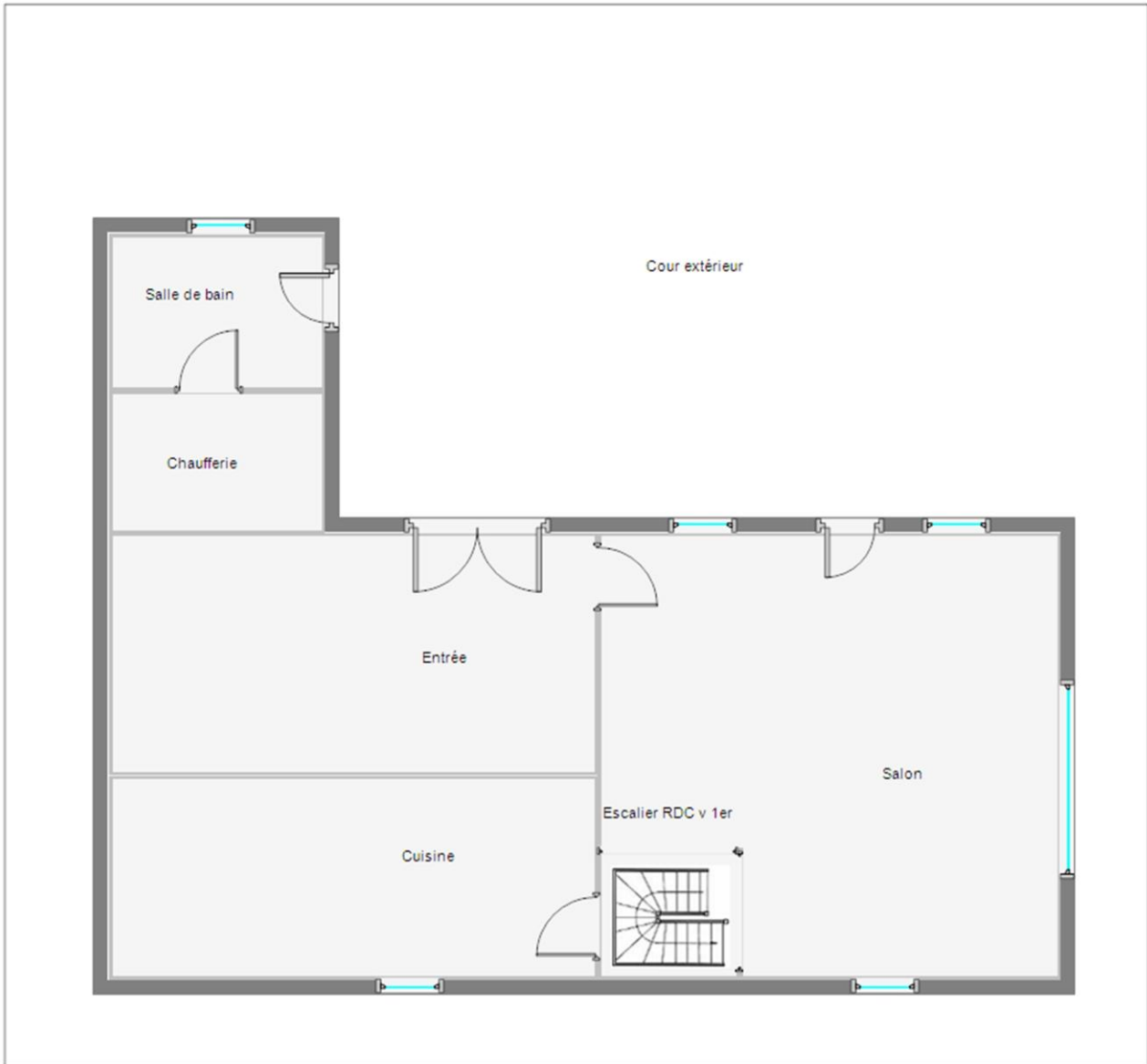
M. FABELS Maison - Blanzaguet 46200 PINSAC Niveau 0
